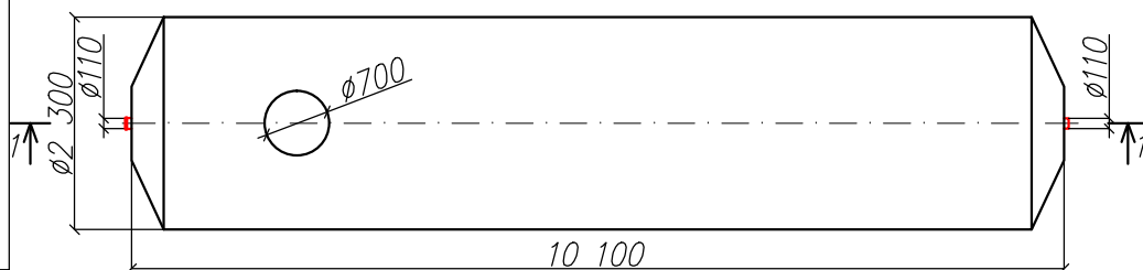
Вид сверху
