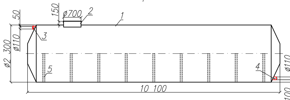
Разрез 1-1
