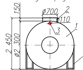
Вид спереди
